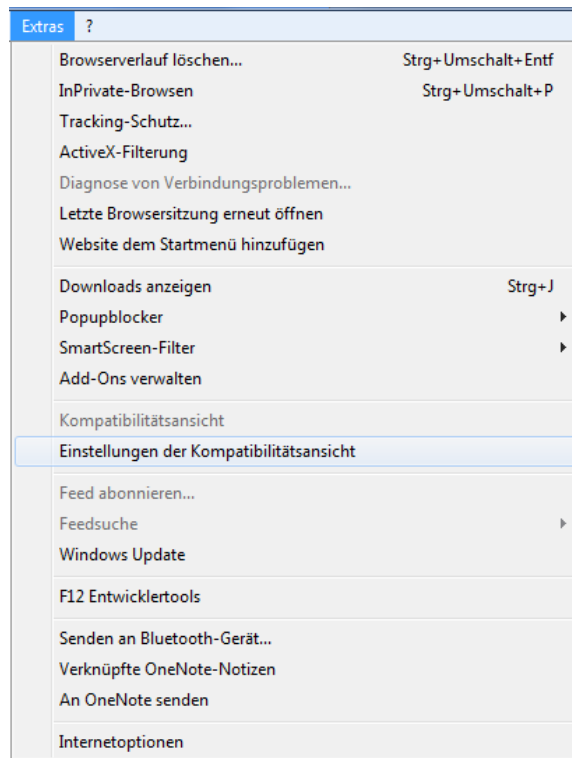
Abbildung 11: Einstellungen Kompatibilitätsansicht
